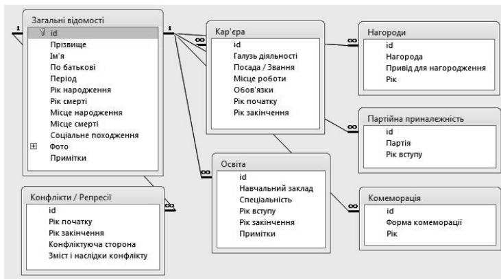
Рис. 1. Структура бази даних «Очільники харківського міського самоврядування».
